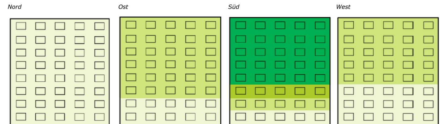
Abb. 37 Jährliches Stromerzeugungspotential und Winterstrom von PV-Fassaden in verschiedenen Orientierungen und Geschossen.
