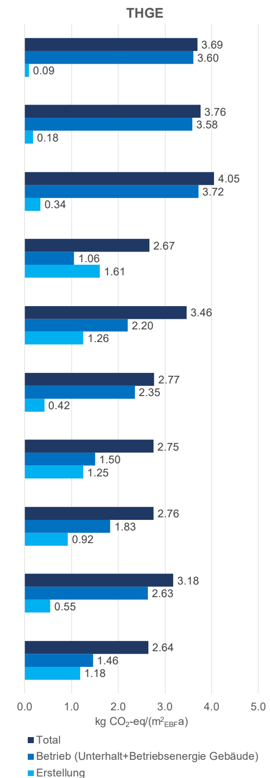
Abb. 56 Treibhausgasemissionen der Referenzfassade (hinterlüftete Fassade mit Faserzementplatten), der verschiedenen Fassadensysteme, der PV-Dachanlage inkl. Referenzfassade sowie die vier Szenarien. Dargestellt sind die Ergebnisse für das Referenzgebäude «Neubau».
