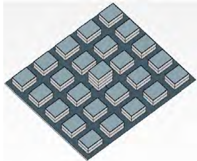
Abb. 47 Simulationsmodell des Gebäudes inkl. Umgebung
