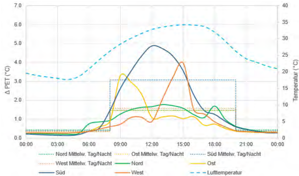
Abb. 50 Einfluss der wandgebundenen Begrünung auf die PET in 1 m Abstand zur Fassade. Dargestellt ist die PET-Differenz im Vergleich zur Referenzfassade an einem sonnigen Sommertag (Hitzetag). Annahme Wind: 1 m/s, Windrichtung: Nord -> Süd.
