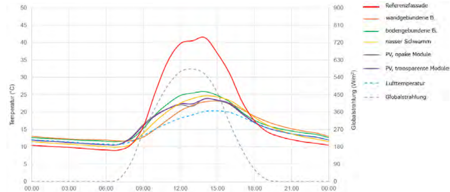
Abb. 44 Temperaturen an der Gebäudefassade (hinter den Fassadenprototypen) an einem milden, sonnigen Tag.
