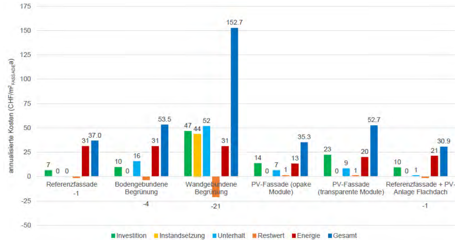
Abb. 40 Annualisierte Kosten (Barwert) der fünf untersuchten Fassadensysteme und der PV-Dachanlage über einen Betrachtungszeitraum von 30 Jahren, dargestellt sind die Ergebnisse für das Referenzgebäude «Neubau».
