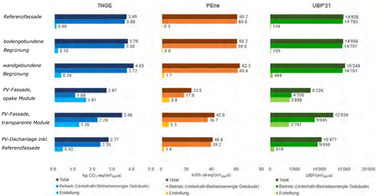
Abb. 38 Treibhausgasemissionen (links), nicht erneuerbare Primärenergie (Mitte) und Umweltbelastungspunkte (rechts) der Referenzfassade, der verschiedenen Fassadensysteme sowie der PV-Dachanlage (inkl. Referenzfassade). Dargestellt sind die Ergebnisse für den achtgeschossigen Neubau. Betrachtungszeitraum: 30 Jahre.
