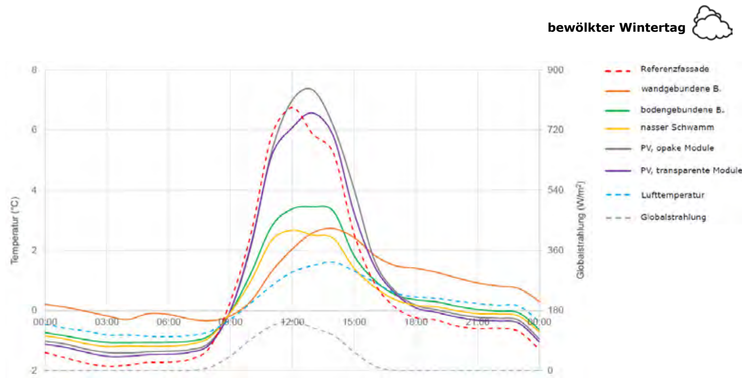
Abb. 45 Oberflächentemperaturen an der Messreferenzfassade und den Fassadenprototypen an einem bewölkten Wintertag.
