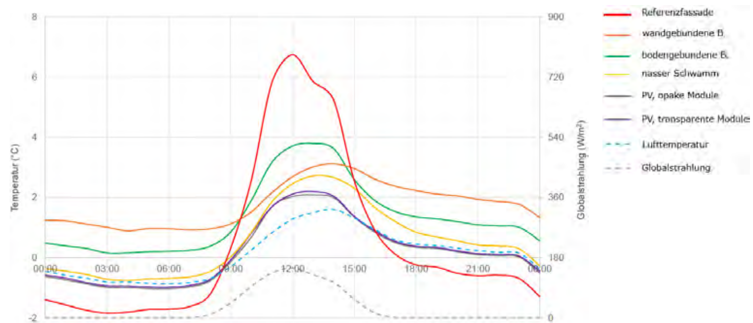
Abb. 46 Temperaturen an der Gebäudefassade (hinter den Fassadenprototypen) an einem bewölkten Wintertag.
