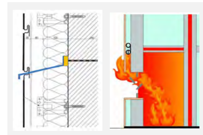
Abb. 66 Bauliche Massnahmen, um im Brandfall die vertikale Ausbreitung von Feuer zu verhindern: Metallprofile (links) oder belüftete Hohlraumabschottungen (rechts). (© Solarwall, Pierre-Olivier Cuche)
