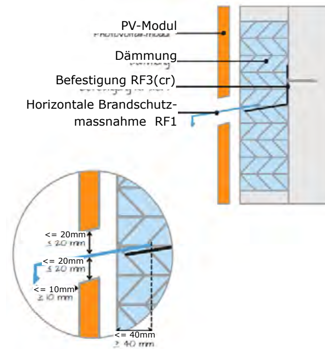
Abb. 118 Schematische Darstellung einer horizontalen Brandabschottung durch ein mit Mineralwolle befülltes Chromnickelstahlelement (© GVB, verändert)
