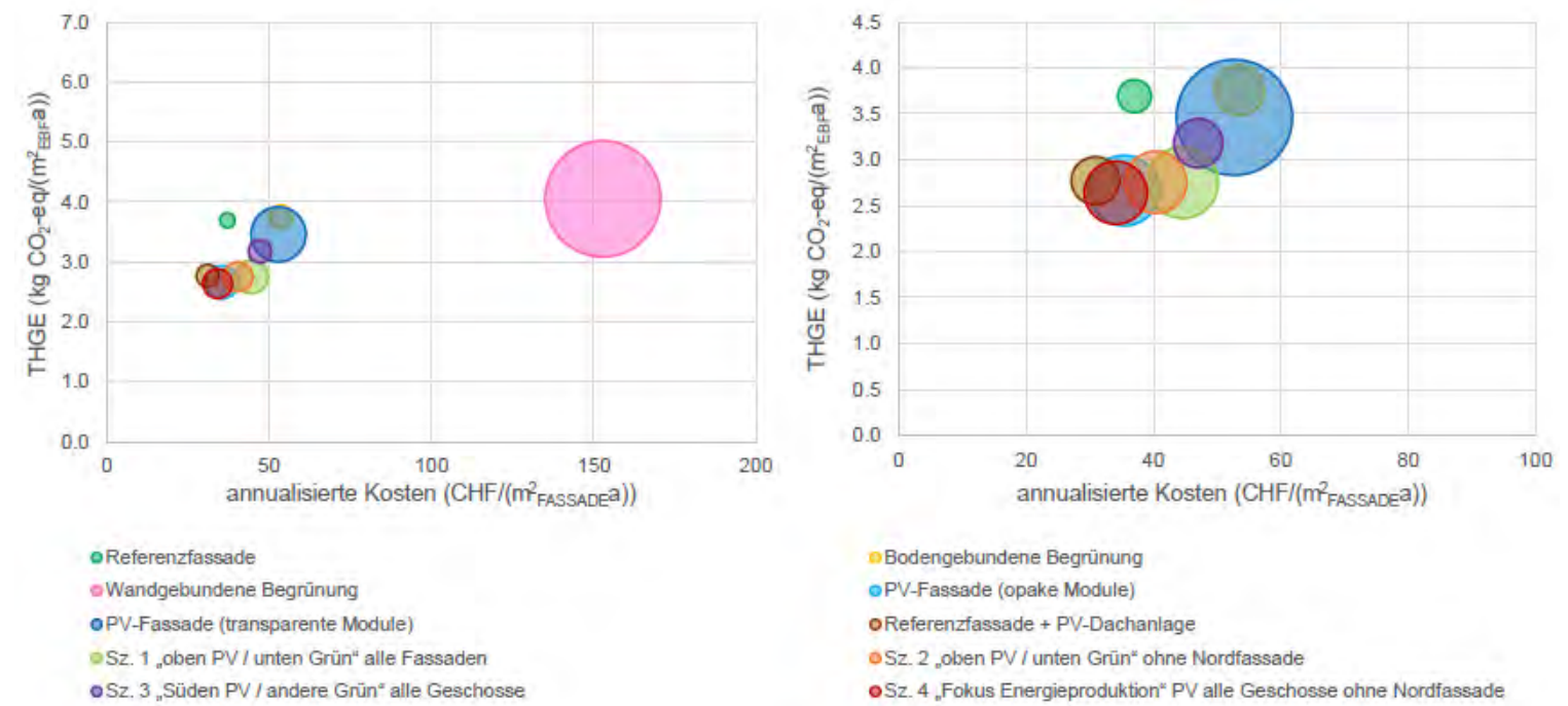
Abb. 58 THGE und annualisierte Kosten während der 30-jährigen Betrachtungsperiode (links: alle Varianten; rechts: vergrößerte Darstellung ohne die wandgebundene Begrünung). Die Grösse des Kreises zeigt die Investitionskosten. Dargestellt sind die Ergebnisse für das Referenzgebäude «Neubau».
