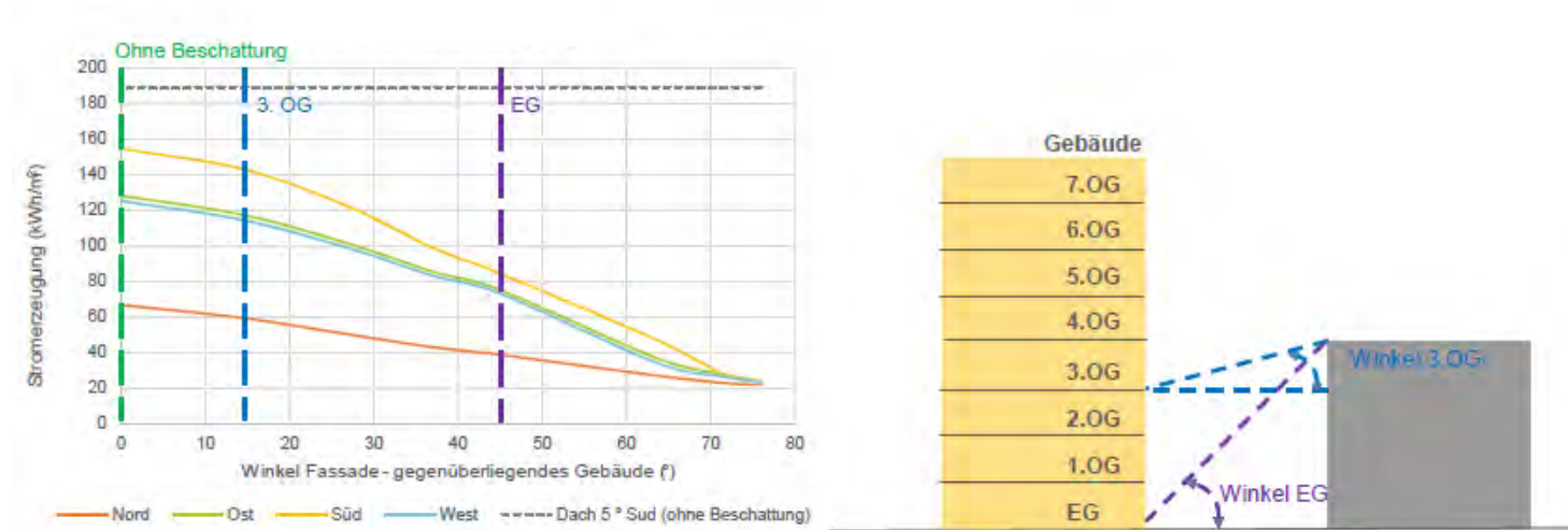
Abb. 34 Jährliche Stromerzeugung in kWh/m 2 an einer Fassade (vertikale Fläche, 90°) in den vier Ausrichtungen Nord, Ost, Süd und West. Eine Verschattung durch Nachbargebäude wurde mitberücksichtigt und wurde durch den Winkel zwischen den beiden Gebäudefassaden dargestellt (die blau-gestrichelte Linie stellt die saisonale Stromerzeugung im 3. OG und die lila-gestrichelte Linie die im EG dar, Annahme: beide Fassaden sind parallel zueinander). Zum Vergleich wurde ebenso die jährliche Stromerzeugung über ein Flachdach mit nach Süden ausgerichteten Modulen mit einem Winkel von 5° dargestellt (grau-gestrichelte Linie)
