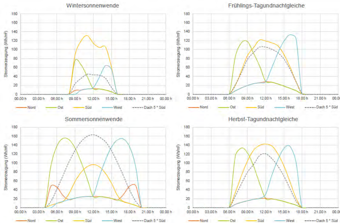
Abb. 36 Stromerzeugungspotential im Tagesverlauf in Wh/m 2 an einer Fassade (vertikale Fläche, 90 °) in den vier Ausrichtungen Nord, Ost, Süd und West ohne Verschattung (Kontext / Nachbargebäude wurden nicht mitberücksichtigt). Dargestellt sind vier Zeiten des Jahres, dazu gehört der Zeitraum um die Wintersonnenwende, die Frühlings-Tagundnachtgleiche, die Sommersonnenwende und die Herbst-Tagundnachtgleiche. Zum Vergleich wurde ebenso ein Flachdach mit nach Süden ausgerichteten PV-Modulen mit einem Winkel von 5 ° dargestellt.
