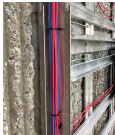
Abb. 115 Kabelkanäle aus feuerfestem Metall (Stahl verzinkt oder CNS) und vertikale Schienen der Unterkonstruktion, auf welchen die Module befestigt werden. Die Kabelkanäle dienen auch zur Brandabschottung. (© Silvia Domingo Irigoyen)
