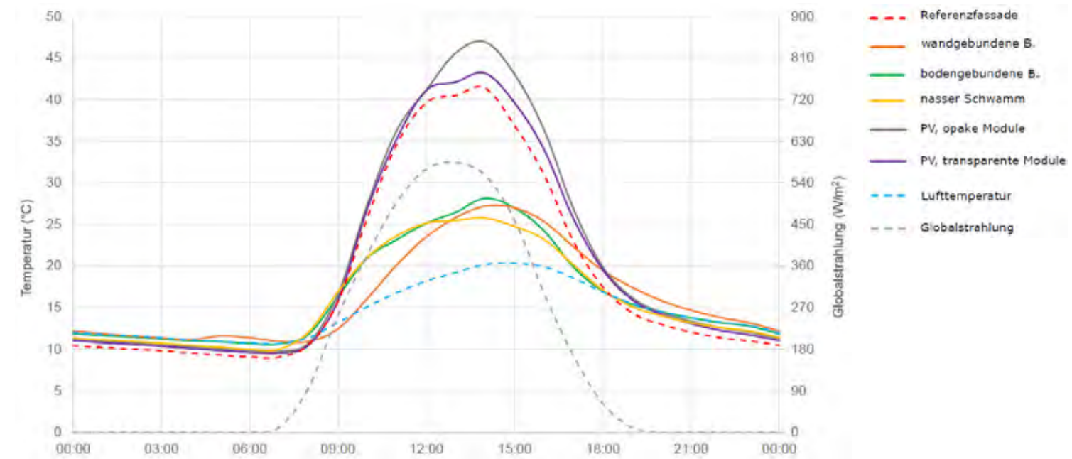
Abb. 43 Oberflächentemperaturen an der Messreferenzfassade und den Fassadenprototypen an einem milden, sonnigen Tag.
