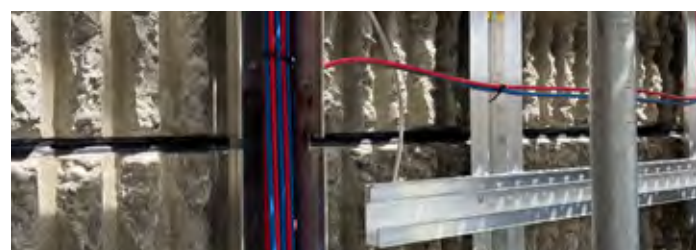
Abb. 1116 Horizontale Elementfuge zwischen den vorgehängten Betonelementen der Fassade (© Silvia Domingo Irigoyen)
