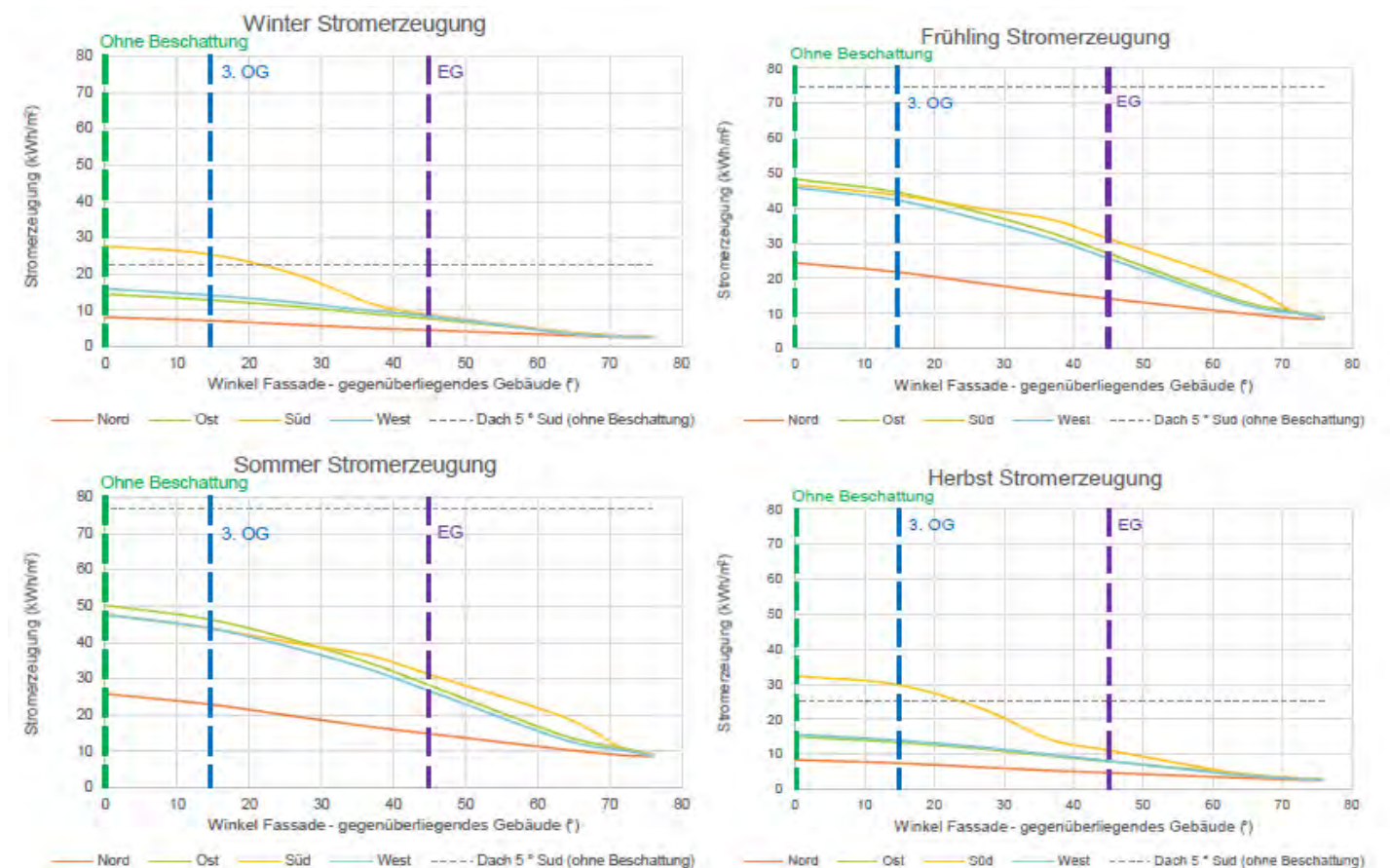
Abb. 35 Saisonale Stromerzeugung in kWh/m 2 an einer Fassade (vertikale Fläche, 90°) in den vier Ausrichtungen Nord, Ost, Süd und West. Eine Verschattung durch Nachbargebäude wurde mitberücksichtigt und wurde durch den Winkel zwischen den beiden Gebäudefassaden dargestellt (die blau-gestrichelte Linie stellt die saisonale Stromerzeugung im 3. OG und die lila-gestrichelte Linie die im EG dar, Annahme: beide Fassaden sind parallel zueinander). Zum Vergleich wurde ebenso die jährliche Stromerzeugung über ein Flachdach mit nach Süden ausgerichteten Modulen mit einem Winkel von 5° dargestellt (grau-gestrichelte Linie).
