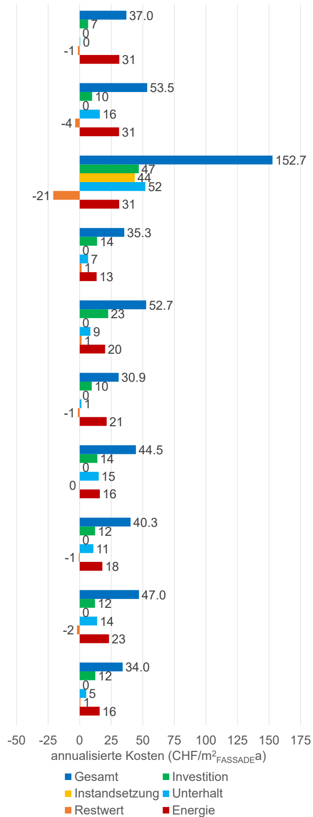
Abb. 57 Annualisierte Kosten (Barwert) der Referenzfassade (hinterlüftete Fassade mit Faserzementplatten), der verschiedenen Fassadensysteme, der PV-Dachanlage inkl. Referenzfassade sowie die vier Szenarien. Dargestellt sind die Ergebnisse für einen Betrachtungszeitraum von 30 Jahren für das Referenzgebäude «Neubau».
