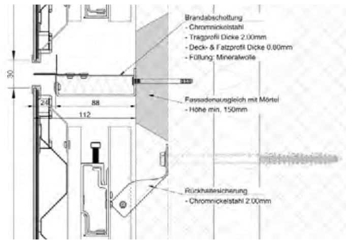
Abb. 1127 Technische Zeichnung der vertikalen Brandabschottung (© Swiss Fassaden Technik AG)
