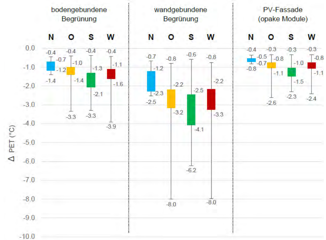
Abb. 49 Einfluss der verschiedenen Fassadensysteme auf die PET an einem Messpunkt in 1 m Abstand zur Fassade. Dargestellt ist die PET-Differenz im Vergleich zur Referenzfassade an einem sonnigen Sommertag (Hitzetag) in den verschiedenen Orientierungen. Die schwarze Linie zeigt die Minimal- und Maximalwerte, welche im Tagesverlauf erreicht werden. Die Balken zeigen den Tages-Mittelwert. Annahme Wind: 1 m/s in «günstiger» und «ungünstiger» Windrichtung.
